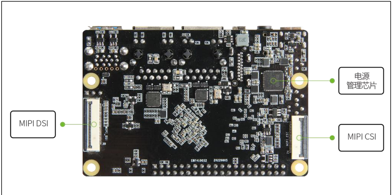
图 4.1-3 鲁班猫 1N 背面视图
