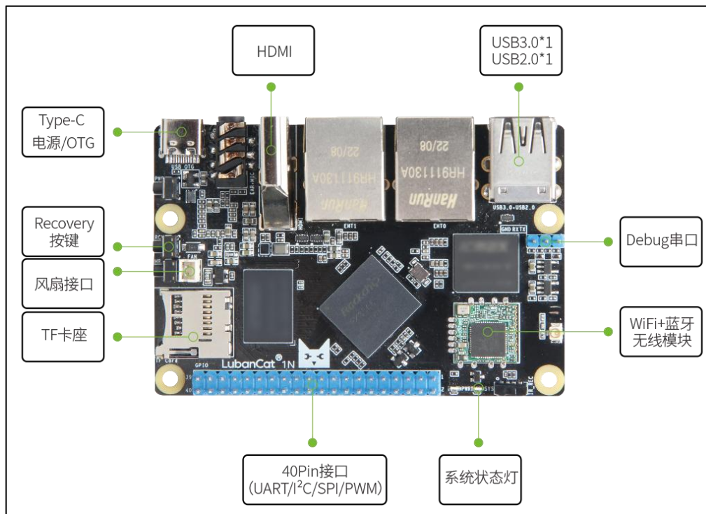
图 4.1-1 鲁班猫 1N 正面视图 1
